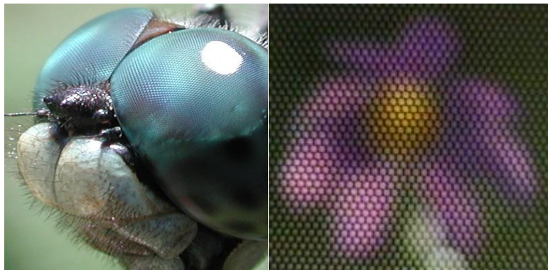
Složené oči hmyzu a mozaikový obraz květiny
